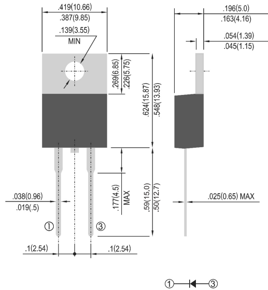
TO-220AC Unit:inch(mm)
